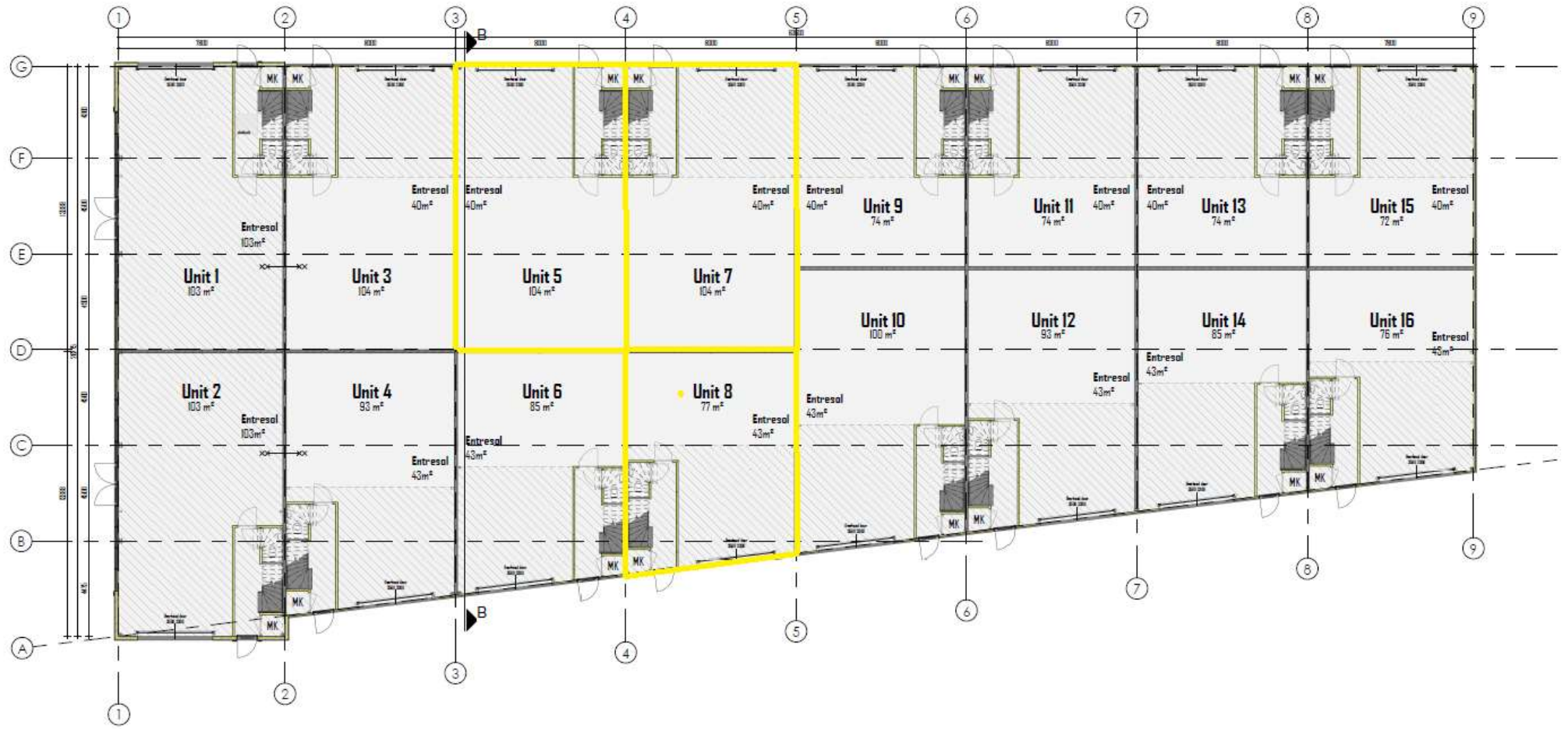
PLATTEGROND
